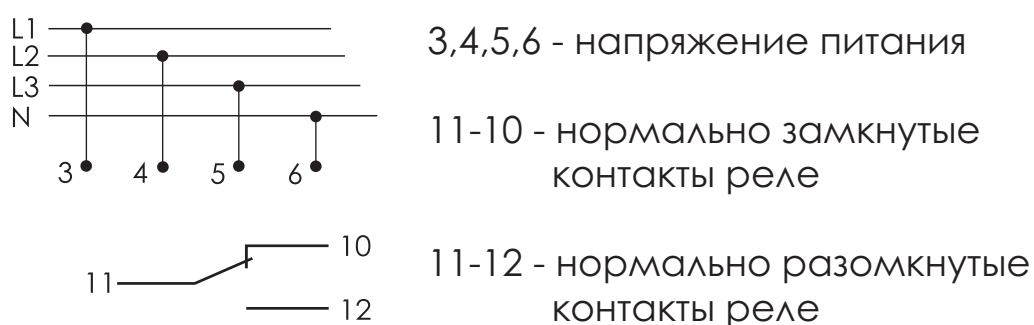
Рис.2 Назначение контактов.
