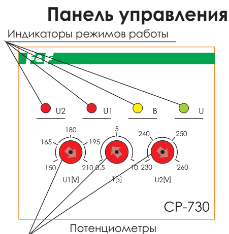
Рис.1 Расположение органов индикации и регулировки.
